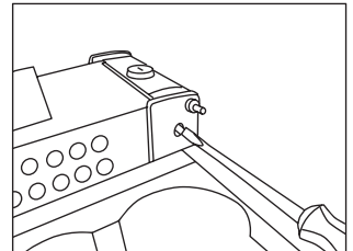
6. Låstappen skruvas fri me
