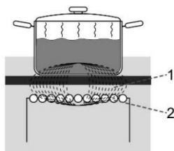
1. magnetfält 2. induktionsrör
